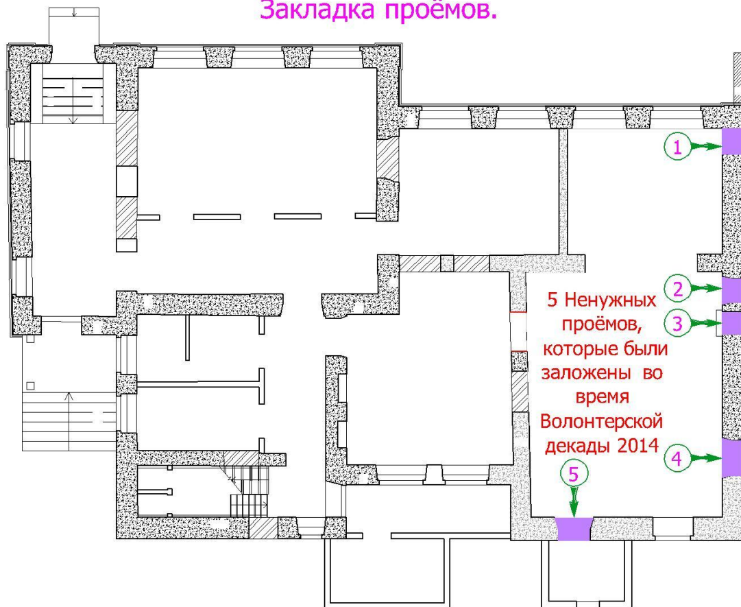
#7. План 1-го этажа с указанием мест закладываемых проемов
